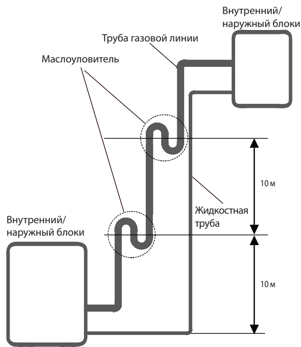
Внутренний блок расположен над наружным
